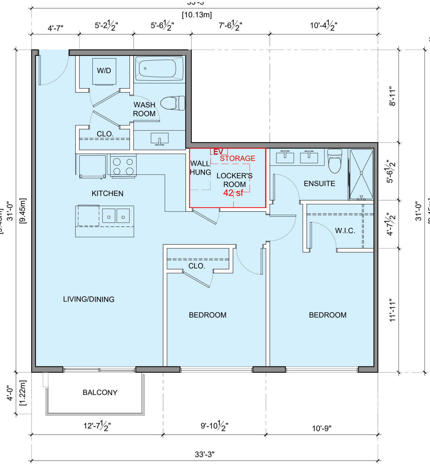
2 UNIT-D 3/16"=1'-0"
