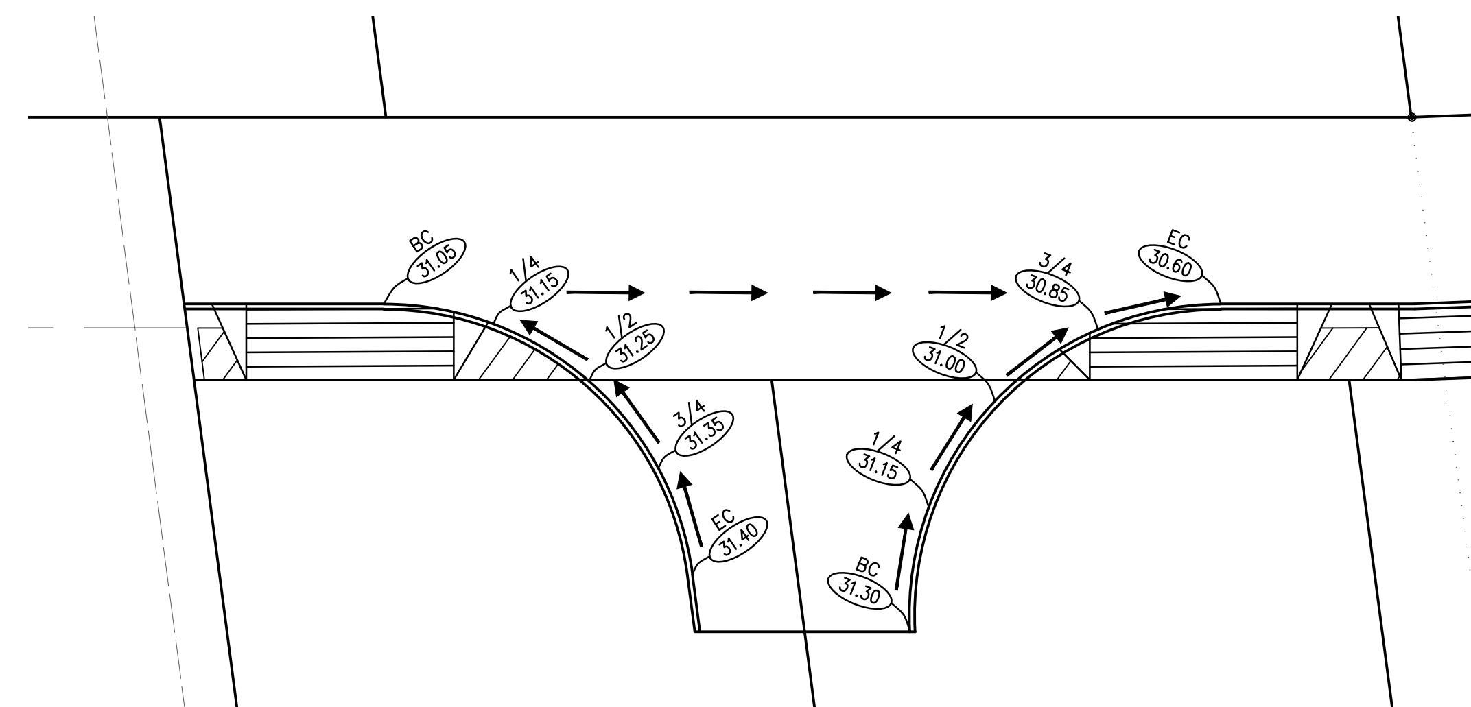
CURB RETURN DETAIL N.T.S.
